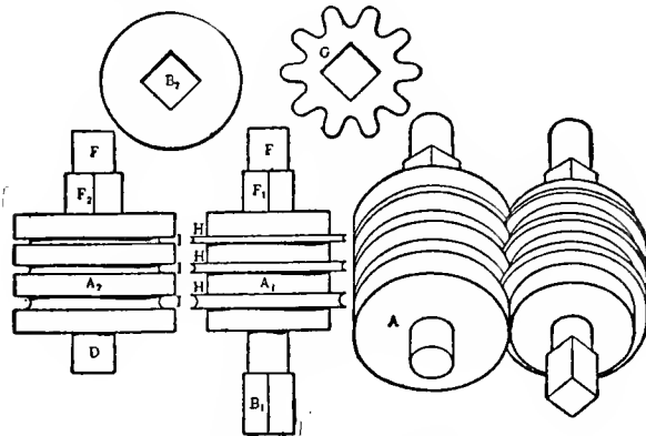
FIG. 14. PURNELL'S ROLLS
